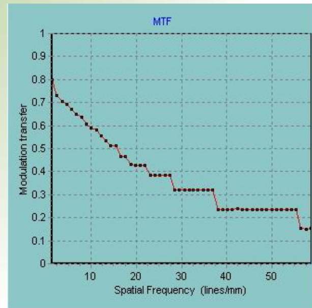
階梯型之有誤差的MTF曲線圖
