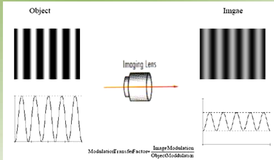
影像輸出入關係圖
