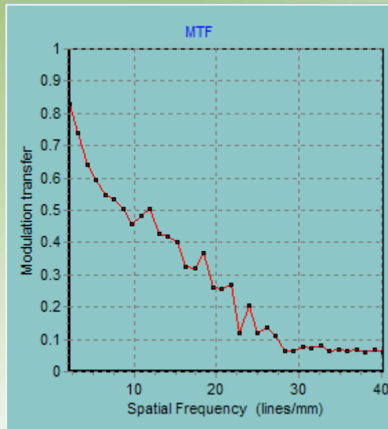
帶著鋸齒狀之有誤差的MTF曲線圖
